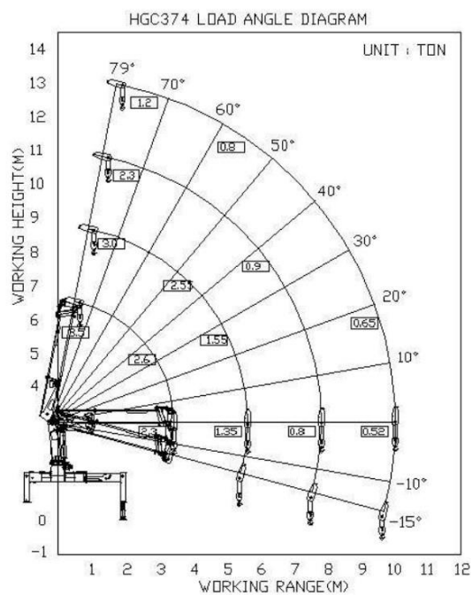
Рис. 2 Диаграмма высотных характеристик КМУ модели HGC374
